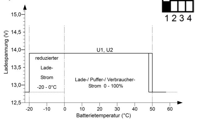
d) LiFePO4 13,9 V
