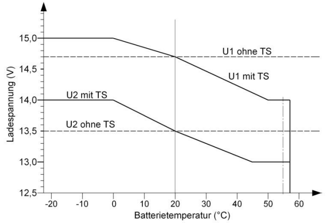
Ladeprogramm „AGM / Vlies“, Kennlinie IU1oU2
