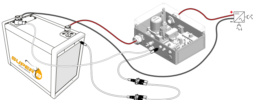
Figure 7. Een Li-ion accu op de SB BIB aansluiten
