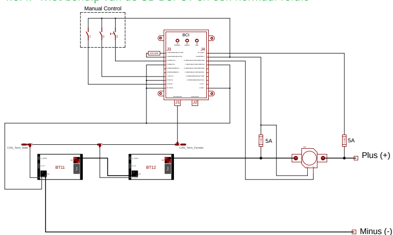
Figure 8. Een Li-ion accu op de SB BCI-C1 aansluiten
